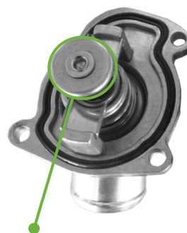
OE termostat (průměr: 22-23 mm)
