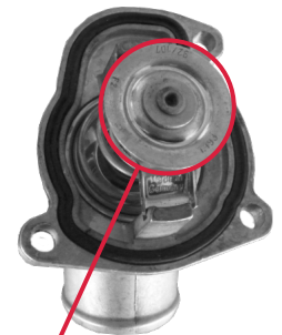
Druhovýrobní termostaty nesplňující OE specifikace (průměr: >23 mm)
