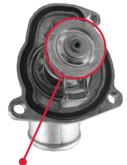
Egyéb alkatrészpiacon található termosztát verzió nem követi a gyári előírásokat (Átmérő >23mm)
