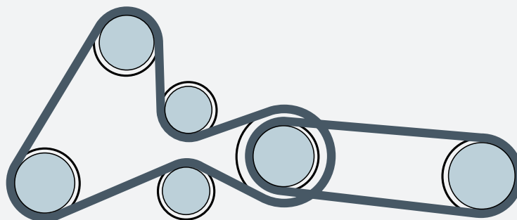
Afb. 2 - Schema secundaire aandrijving (vanaf motor nr. 0113090), uitgerust met de elastische multi-V-riem 40717.
