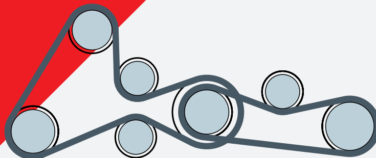
Afb. 1 - Schema secundaire aandrijving (tot en met motor nr. 0113089), uitgerust met spanrol 30167 en multi-V-riem 28798.
