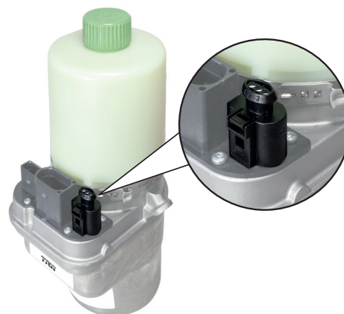
Čerpadlo pomocného řízení s uzavíracím konektorem
