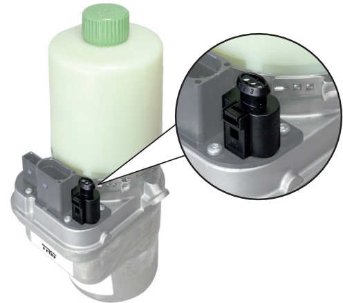
Kapama soketli direksiyon pompası
