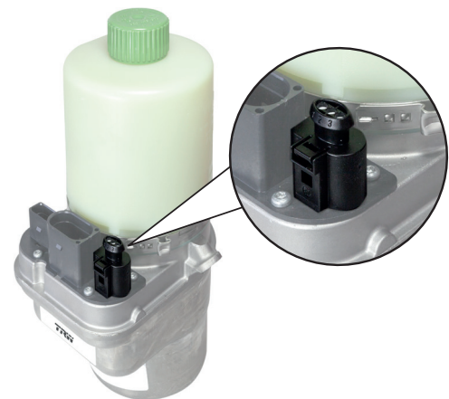
有密封塞的转向助力泵
