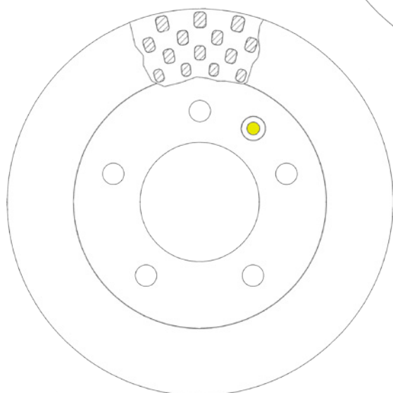
Brzdový kotouč s otvorem pro malé ustalovací šrouby
