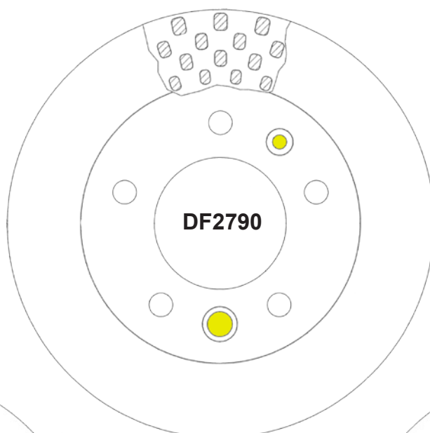
Brzdový kotouč s otvory pro malé a velké ustalovací šrouby
