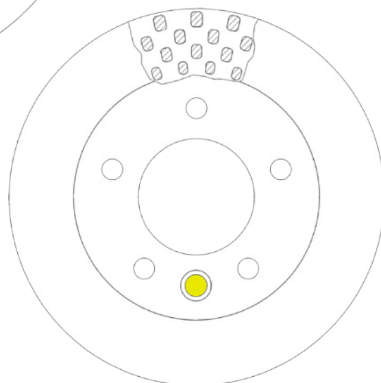
Brzdový kotouč s otvorem pro velké ustalovací šrouby
