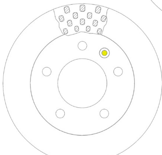
Disco de freno con agujero para tornillos de fijación pequeños
