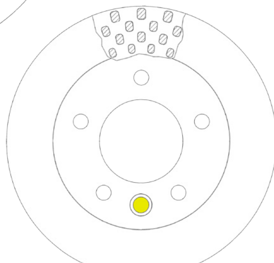
Disco de freno con agujero para tornillos de fijación grandes
