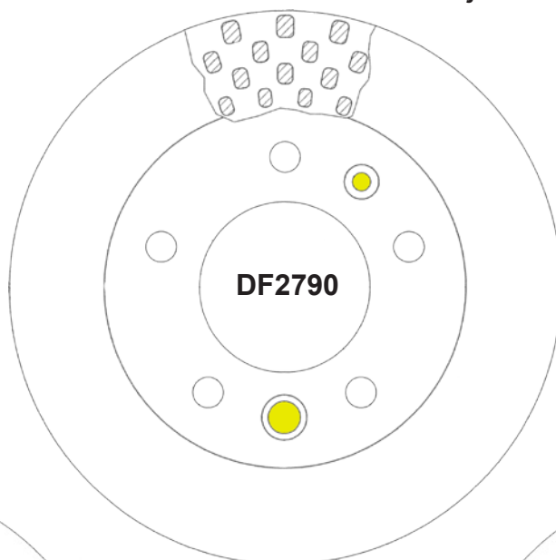
Disco de freno con agujeros para los tornillos de fijación grandes y pequeños
