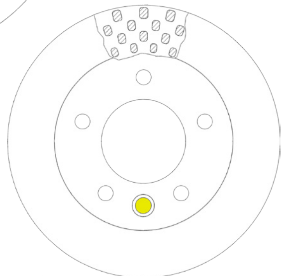
Remschijf met gat voor grote fixeerbouten
