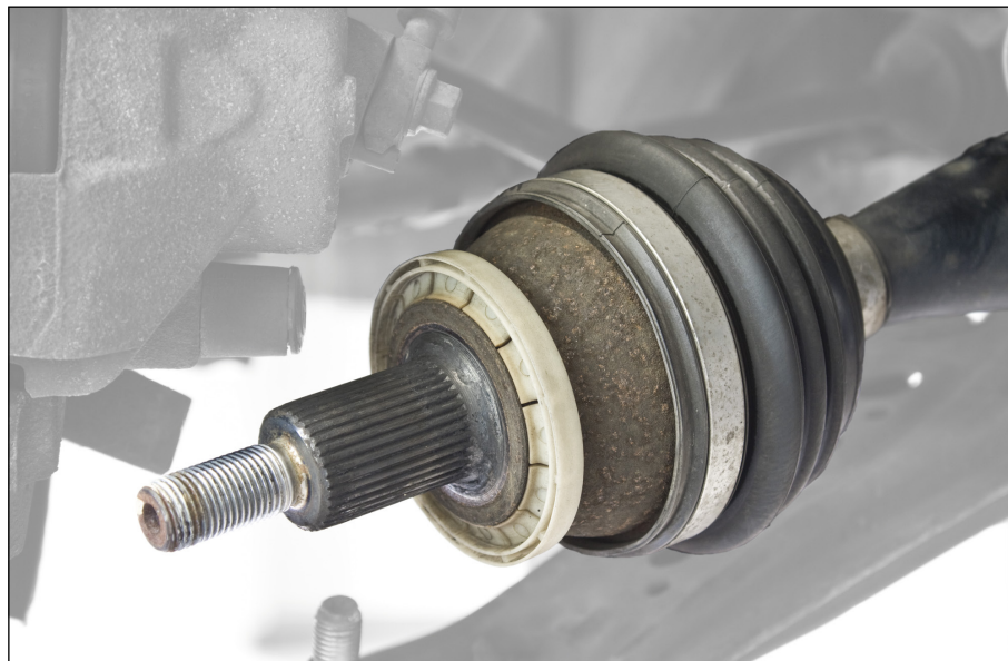
Slika 1: Tesnilni obročki lahko odstopajo v oblikovanju in barvi!
