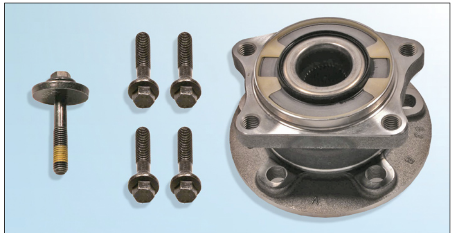
Figura 1: FAG-Kit 713 6186 30
