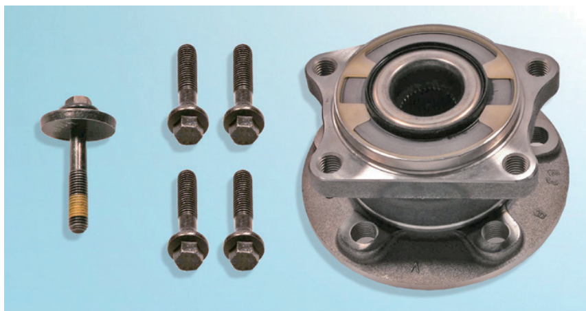
図1：FAG キット 713 6186 30
