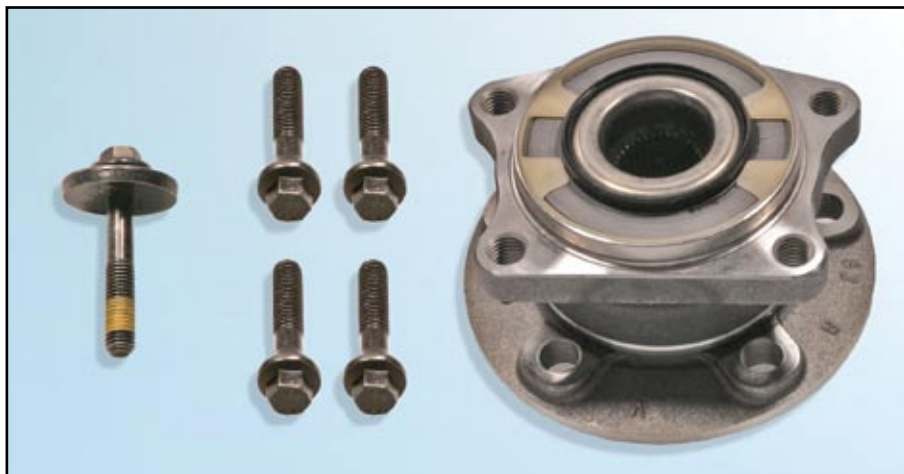
Foto 1: Zestaw łożysk kół FAG KIT 713 61863 0
