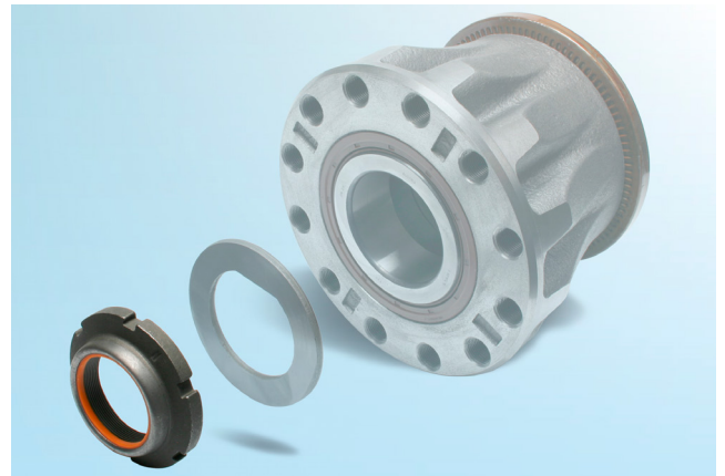
Kuva 1: Akselitapin mutteri 434 0431 10 on saatavana FAG-varusteena
