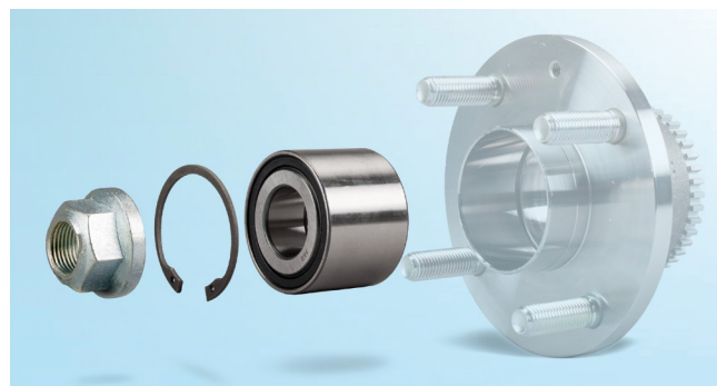
Figur 1: FAG-hjulkulelagersettet 713 6448 00 som en reparasjonsløsning – det er ikke nødvendig å skifte ut hjulnavet.
