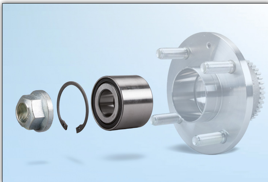
Obrázok 1: FAG súprava ložiska kola 713 6448 00 ako riešenie pre opravy – náboj kola nie je nutné vymieňať.
