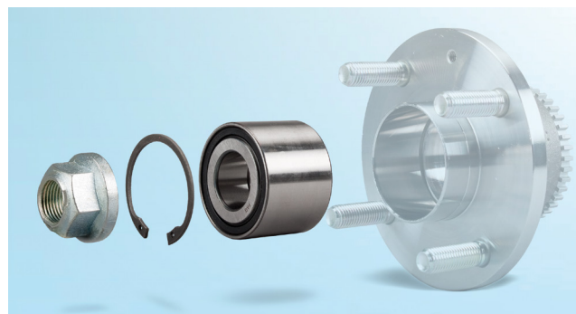
Bild 1: FAG hjullagersats 713 6448 00 som reparationslösning – byte av hjulnav överflödigt.
