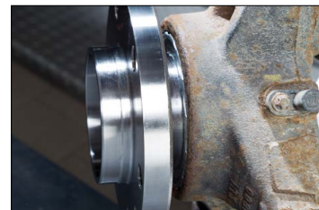
Slika 3: Sigurnosni prsten mora biti poravnat sa rukavcem točka
