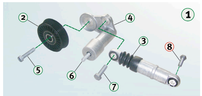
Εικόνα 1: Λεπτομερής περιγραφή του 534 0014 10 με όλα τα εξαρτήματα
