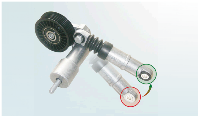
Εικόνα 2: 534 0014 10 - Παραλλαγή με λευκά και μαύρα πλαστικά μάτια στον υδρ. αποσβεστήρα
