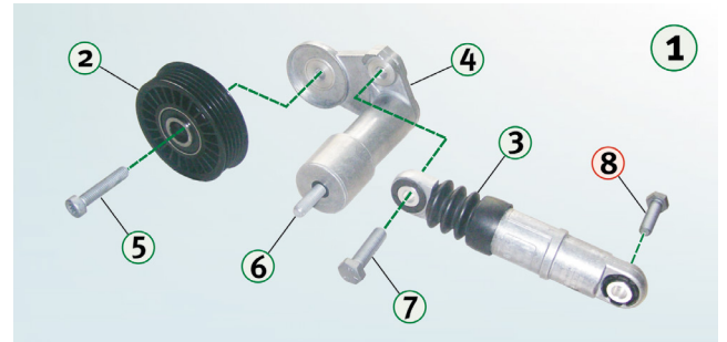
Kuva 1: Yksityiskohtaisesti esitetty 534 0014 10 kaikkine osineen
