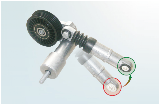
Kuva 2: 534 0014 10 - mallit hydraulivaimentimen kiinnityssilmukkojen valkoisilla ja mustilla muovikoteloilla
