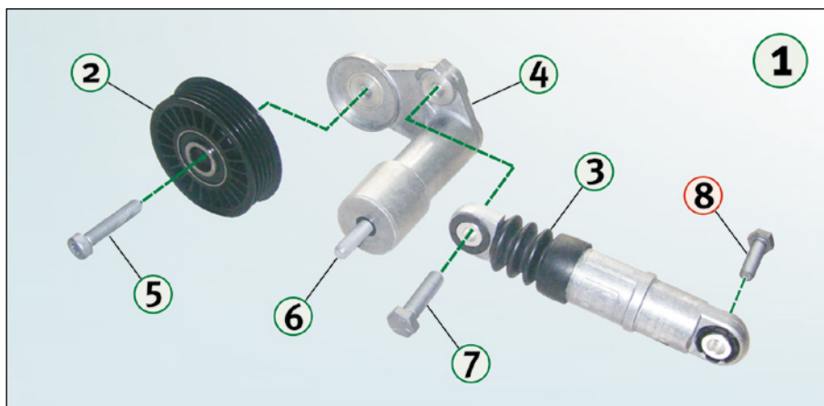
Figura 1: Rappresentazione in dettaglio del 534 0014 10 con tutti i componenti
