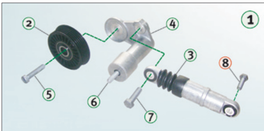
Fig. 1: Detailafbeelding van 534 0014 10 met alle componenten
