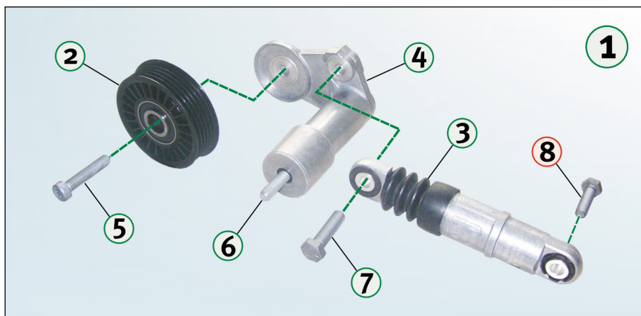
Obrázok 1: Detailné znázornenie 534 0014 10 so všetkými komponentmi
