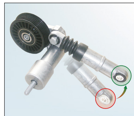
Obrázok 2: 534 0014 10 – vyhotovenie s bielymi a čiernymi plastovými puzdrami upevňovacích ôk hydraulického tlmiča
