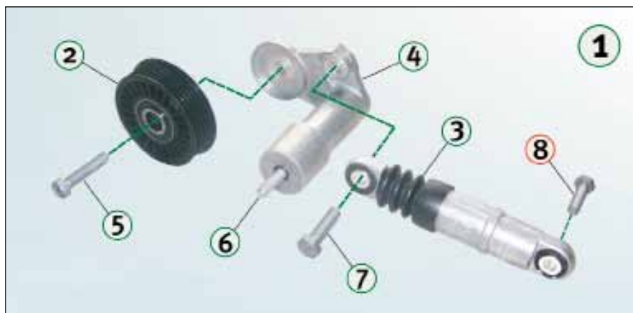
Slika 1: Detajlni prikaz 534 0014 10 z vsemi komponentami
