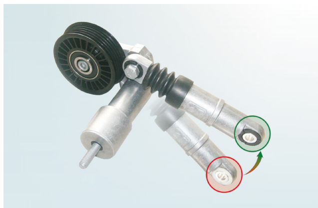
Bild 2: 534 0014 10 – utförande med vita och svarta plastbussningar hos den hydrauliska dämparens fästhål
