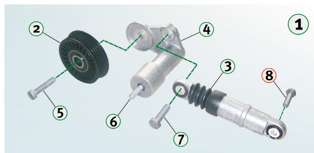
Bild 1: Detaljbild till 534 0014 10 inkluderande samtliga komponenter
