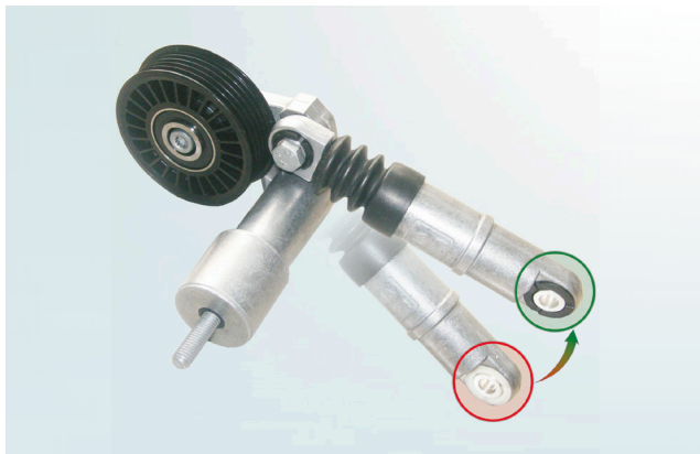
Зображення 2: 534 0014 10 — цей варіант оснащений чорною та білою втулками гідравлічного демпфера
