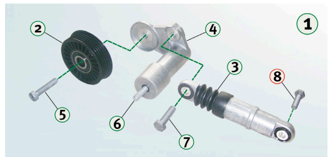
Зображення 1: Детальне зображення вузла 534 0014 10 з усіма компонентами
