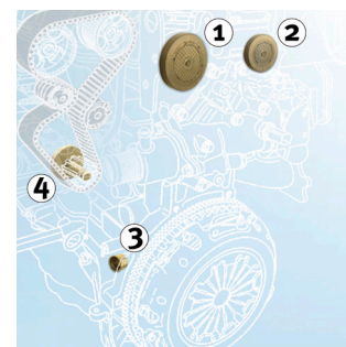
Obr. 2: Montážní pozice
