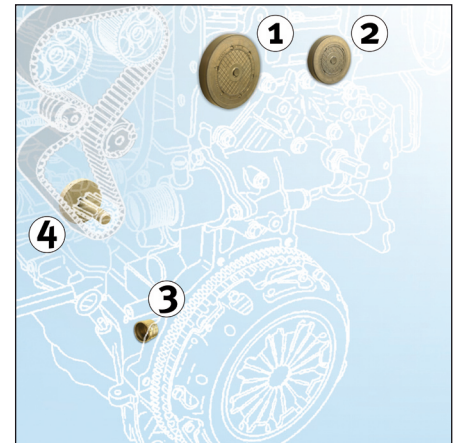
Bild 2: Einbauposition
