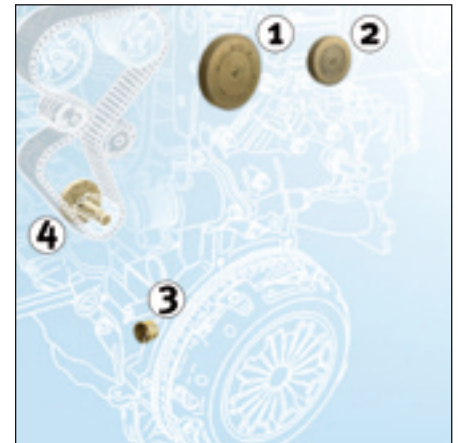
Fig. 2: Inbouwpositie
