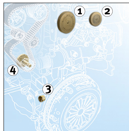
Obr. 2: Montážna pozícia
