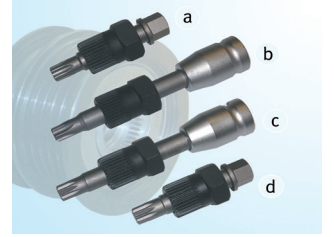
Şekil 4: Özel aletler
