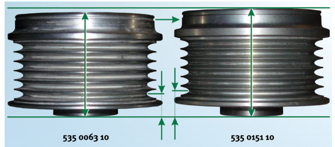
Kuva 3: Laturin vapaapyörrien 535 0063 10 (VALEO) ja 535 0151 10 (DENSO) erot.
