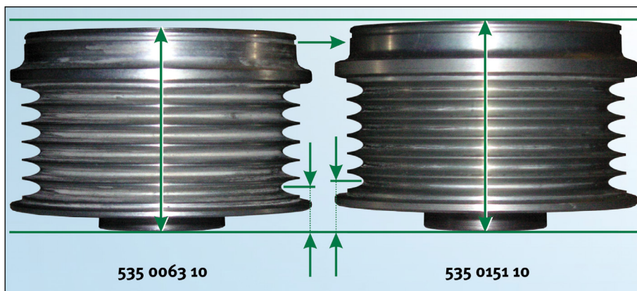
Slika 3: Razlikovanje remenica za slobodni hod alternatora INA 535 0063 10 (VALEO) i 535 0151 10 (DENSO)
