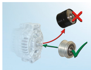
1. ábra: Termékhelyettesítés
