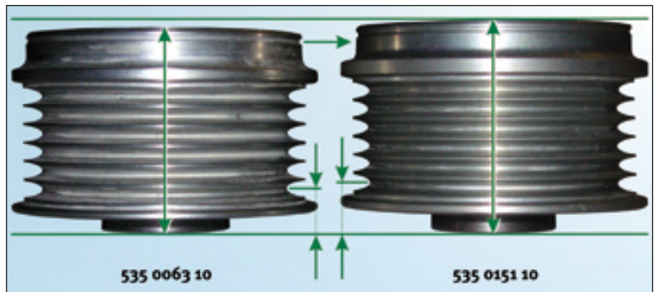
Fig. 3: De INA-generatorvrijlooprollen onderscheiden 535 0063 10 (VALEO) en 535 0151 10 (DENSO)
