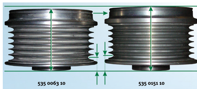
Figur 3: Skille mellom INA-friløpremskive OAP 535 0063 10 (VALEO) og 535 0151 10 (DENSO)
