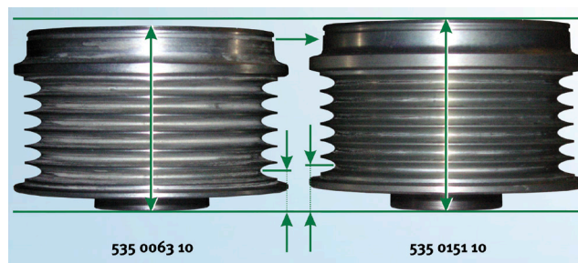
Рисунок 3: Различие между шкивами генератора с обгонной муфтой INA 535 0063 10 (для VALEO) и 535 0151 10 (для DENSO)
