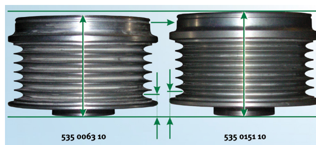
Bild 3: Skillnader hos INA frinavremskivor INA 535 0063 10 (VALEO) och 535 0151 10 (DENSO)
