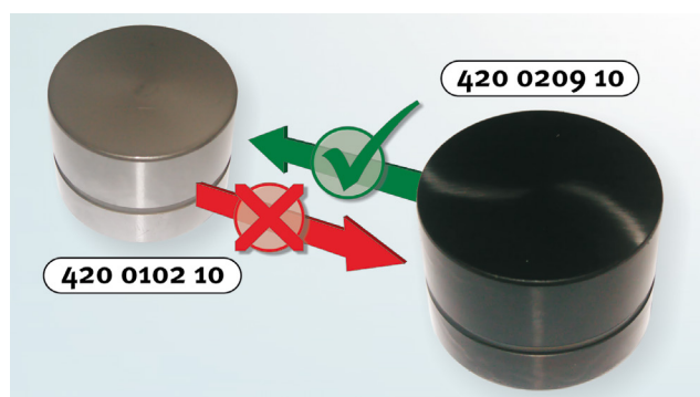
Figur 1: 420 0102 10 kan ikke byttes om med 420 0209 10
