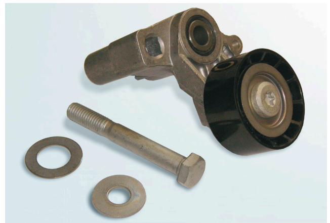
Εικόνα 2: 534 0100 20 – παλιός σχεδιασμός
