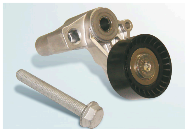
Рисунок 1: 534 0100 20 – текущая конструкция
