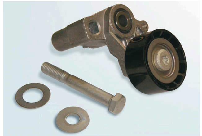
Зображення 2: 534 0100 20 – попередня конструкція
