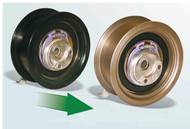
Obrázek 1: Vylepšená povrchová úprava oběžné dráhy – zde znázorněno jako příklad u objednáčho č. 531 0524 30
