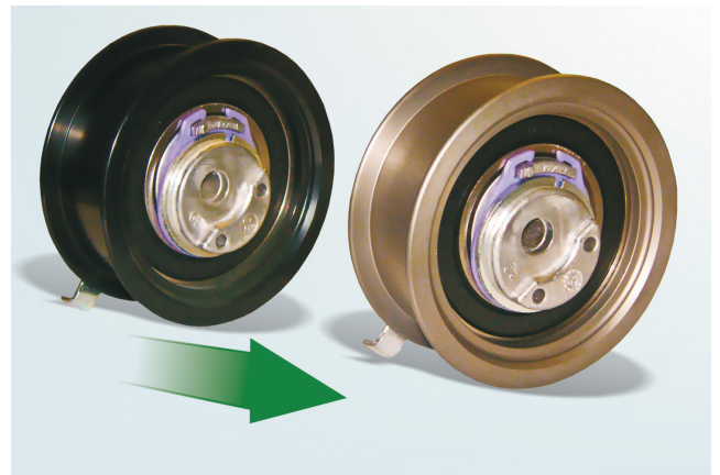
Kuva 1: Esimerkinä hihnankiristin (tuotenro INA. 531 0524 30)
