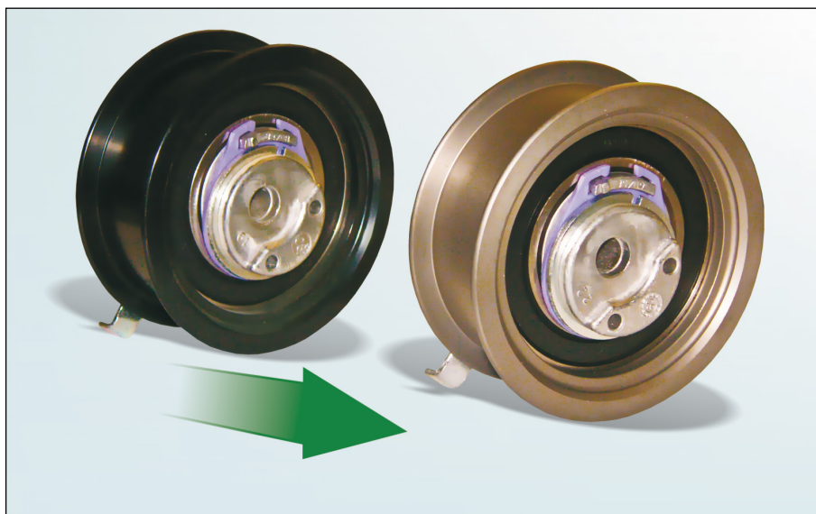
Slika 1: Poboljšana površinska obrada dodirne staze natezne rollice – ovdje prikazano kao primjer za br. artikla 531 0524 30
