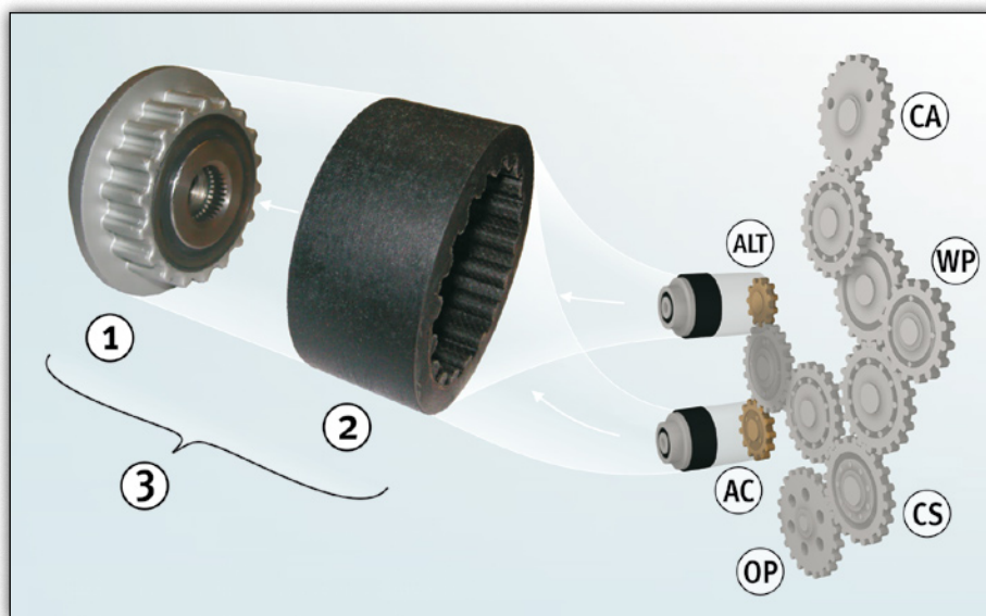
Fig 1: Polea libre del alternador con manguito de acoplamiento flexible y engranaje recto
