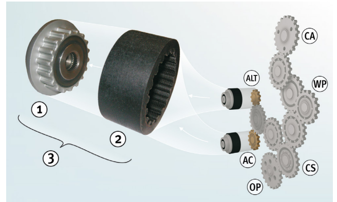
Kuva 1: Laturin vapaapyörä joustavalla liitosholkilla ja sijainnit hammaspyörästä
