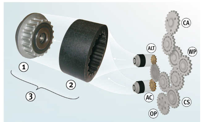
Figur 1: Friløpremskive med fleksibel koplingsmuffe og tanddrev
