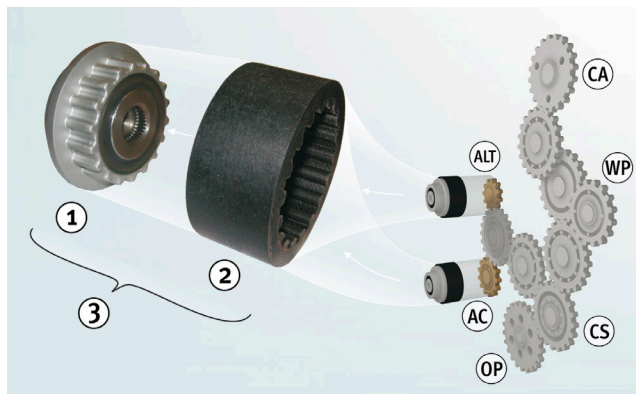
Figura 1: Rolă cu roată liberă pentru alternator cu manșon de cuplare flexibil și roată dințată cilindrică
