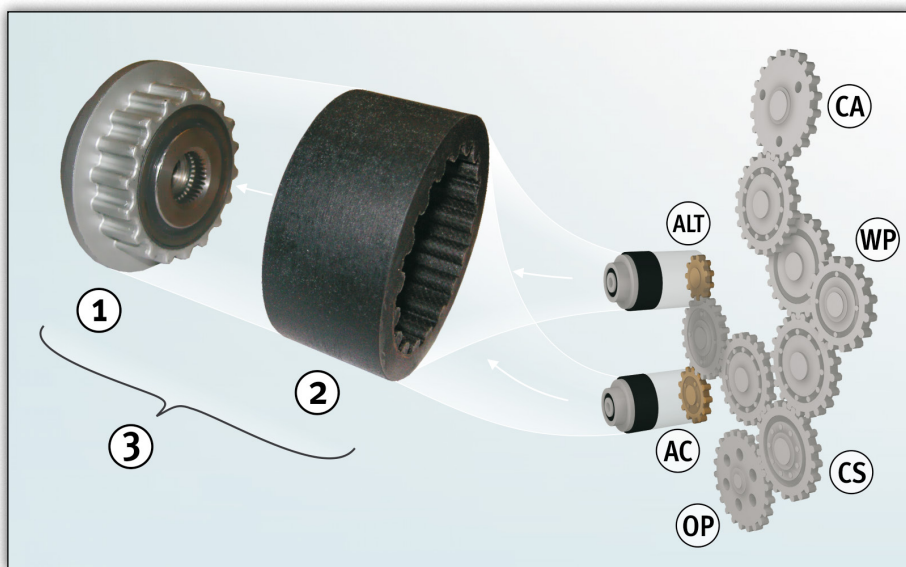
Slika 1: sklopka za prosti tek generatorja s fleksibilno spojno obojko in s pogonom z valjastimi zobniki
